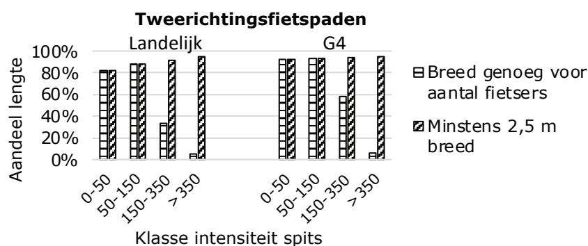
Afbeelding 6. Aandeel van de lengte aan verplichte tweerichtingsfietspaden binnen de bebouwde kom die voldoet aan de eisen voor verhardingsbreedte in de Ontwerpwijzer fietsverkeer (CROW, 2016)
