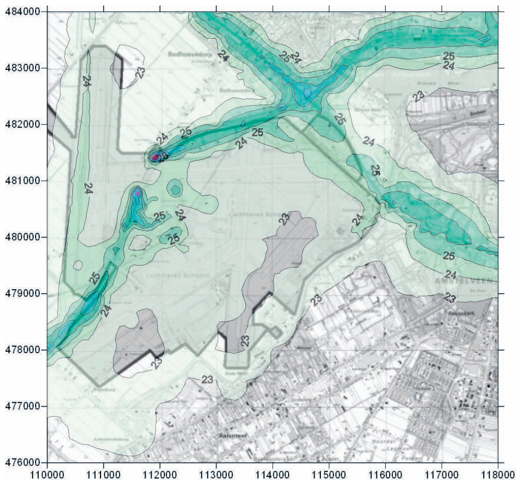
Figuur D.8. Referentiescenario PM_{10} concentraties (in \mu g/m^3 ) voor het jaar 2010 in 8 x 8 km gebied rondom Schiphol
