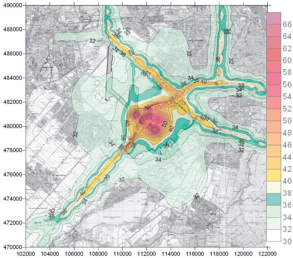
Figuur 2. Planalternatief NO2 concentraties (in µg/m3) in jaar 2010 in 20x 20 km gebied rondom Schiphol
