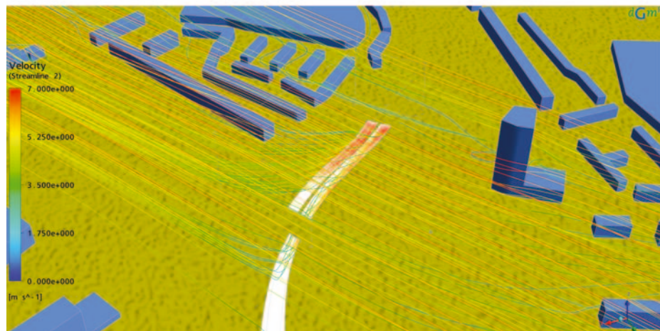
Figuur 29 Voorbeeld van stroomlijnen die inzicht geven in de luchtstromingen in het model
