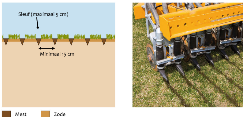
Figuur 2.5.3 Zodebemester, mest komt een paar centimeter diep in de bodem (foto: Veenhuis bv).
