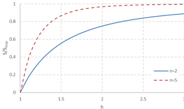
Figuur 3 Relatie tussen sedimentimport en de morfologische toestand. h = 1 vertegenwoordigt het morfologische evenwicht zonder ZSS. De sedimentimport S benadert de maximale waarde voor grote waarden van h . n is een parameter in de formulering voor sedimenttransport en is afhankelijk van de sedimentsoort (zand of slib).
