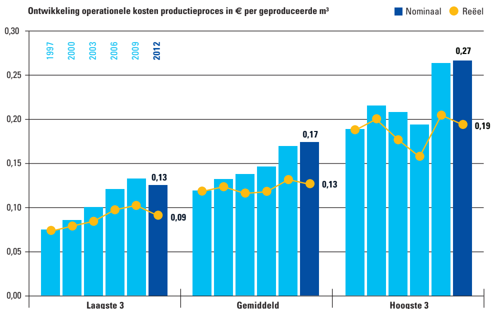
Ontwikkeling operationele kosten productieproces in € per geproduceerde m 3
