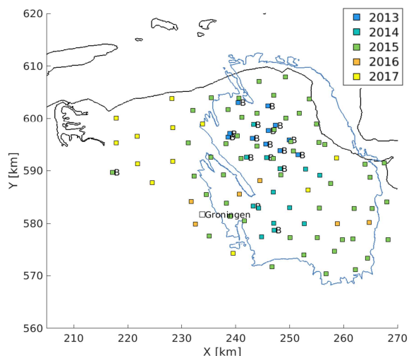
Figuur 1: Het versnellingsmeternetwerk in Groningen
