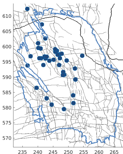
Figuur 2: Aardbevingen met een magnitude van 2,5 en hoger sinds 1991 1
