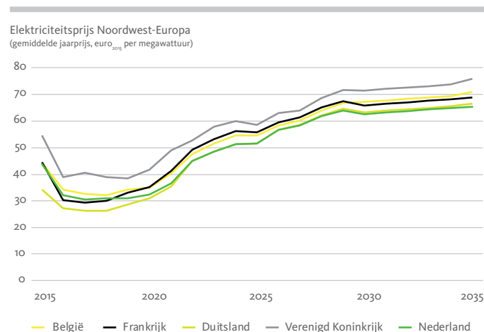
Figuur 2.8 Groothandelsprijs elektriciteit ramingen Noordwest-Europa
