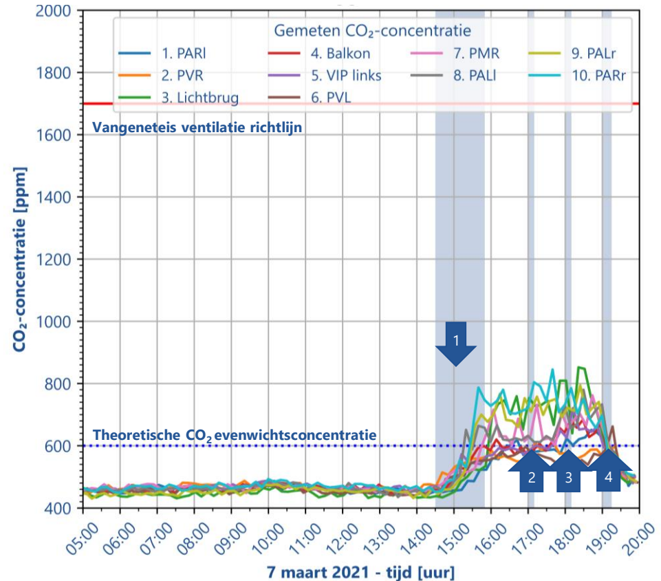
Figuur 6: Verloop CO 2 concentratie tijdens het Concert in de Ziggo Dome.
