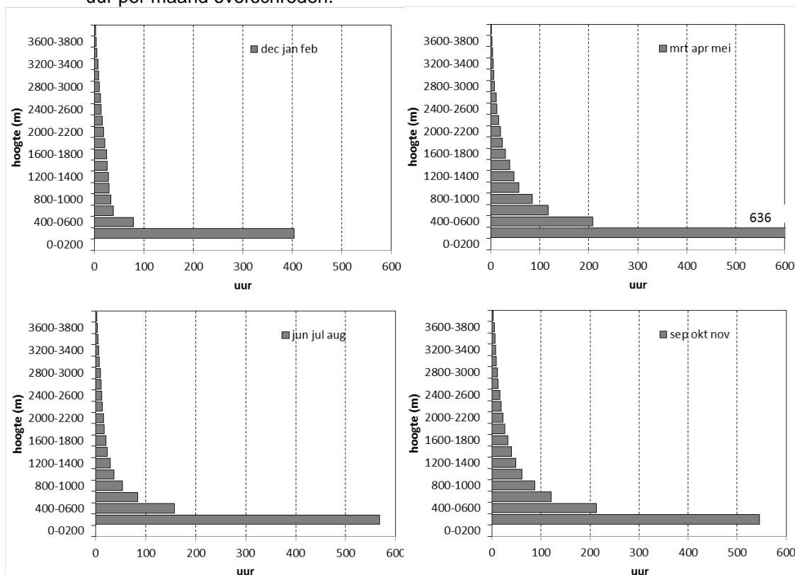
Figuur 3.1 Cumulatieve verdeling van dichtheidsklassen >10 \text{ ex/km}^3 (Birdtam 5, 6, 7 en 8) over de kolom van 200-4.000 m hoogte; uitgedrukt in gemiddeld aantal uren per drie maanden.
