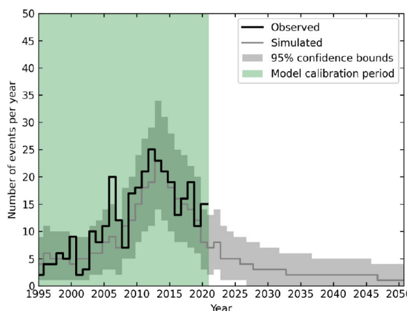
Figuur 3.3 Verwachte seismische activiteit en variatie per gasjaar voor een koud temperatuurverloop. Onderschrift als in Figuur 3.1.
