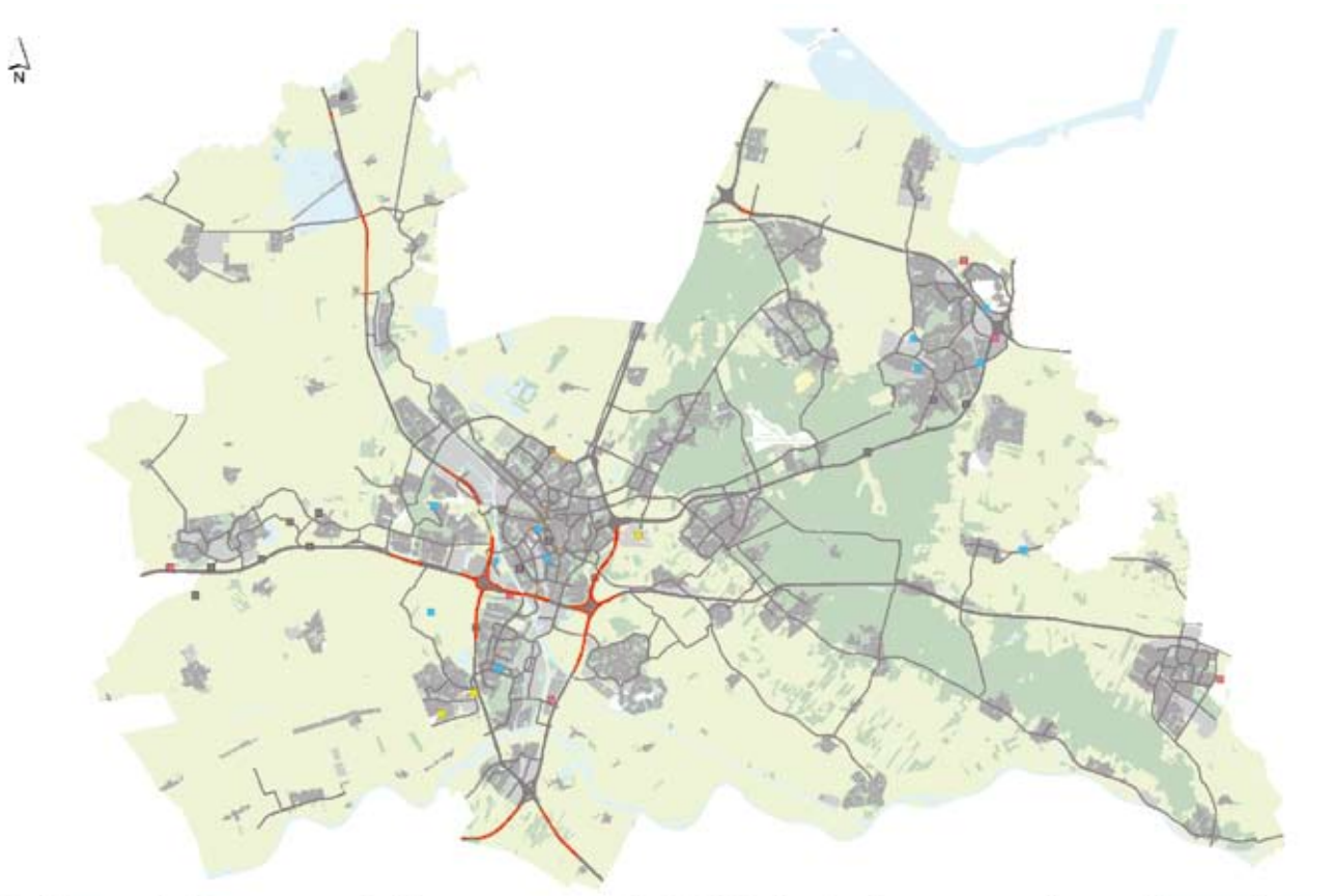
Utrecht, overschrijdingen grenswaarde NO2 in 2015 na generiek rijksbeleid: de regionale restopgave
