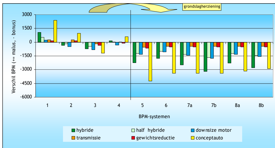
Figuur 2 Verschil in te betalen BPM (t.o.v. de referentietechniek) bij toepassing van verschillende brandstofbesparende technieken bij een benzine-uitvoering van een Opel Astra Stationwagon
