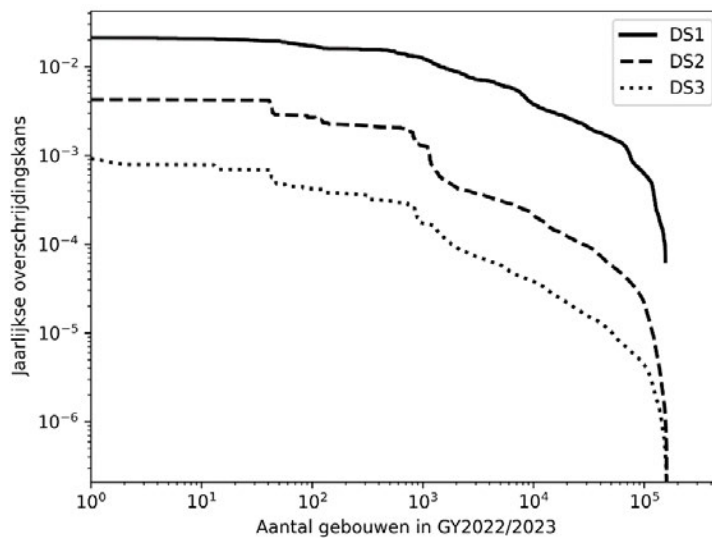
Figuur 6.1: Jaarlijkse overschrijdingskans voor schadetoestanden DS1 t/m DS3 voor gasjaar 2022/2023 voor alle gebouwen samen in de exposure database voor scenario Update maart 2023 .
