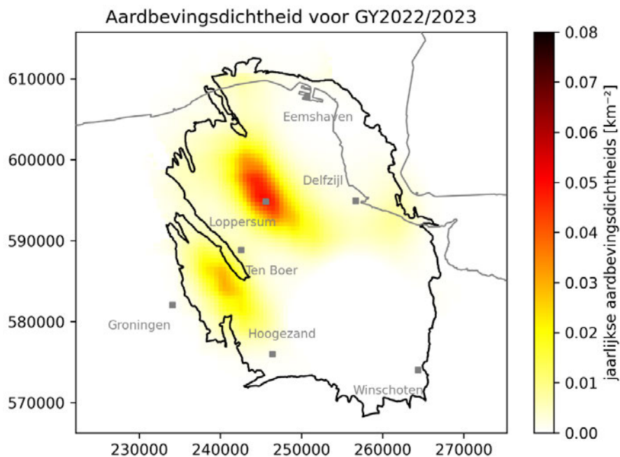
Figuur 3.2: Jaarlijkse aardbevingsdichtheid (aantal aardbevingen per \text{km}^2 ) voor gasjaar 2022/2023 voor scenario Update maart 2023 .
