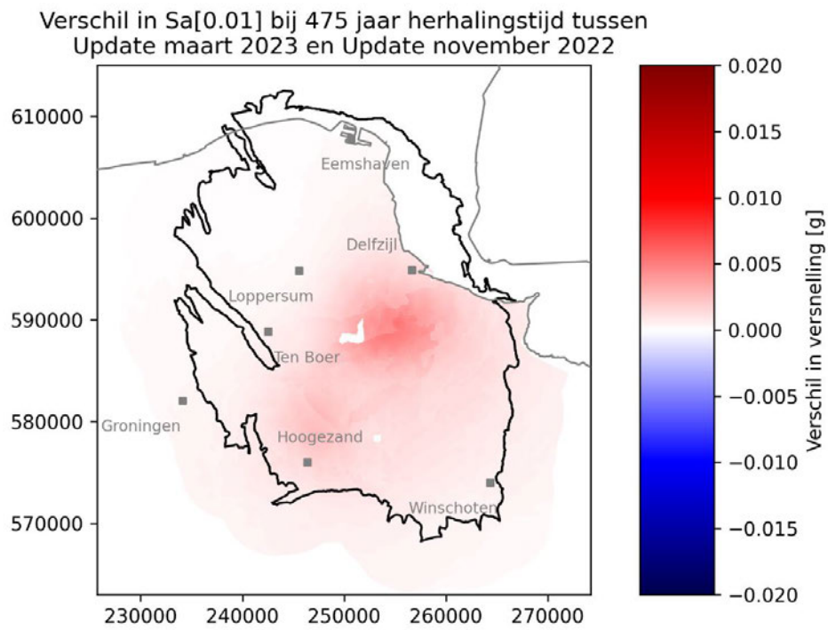
Figuur 4.2: Vershil in verwachte seismische dreiging tussen Update maart 2023 en Update november 2022 (cf. het Vaststellingsbesluit gasjaar 2022/2023).
