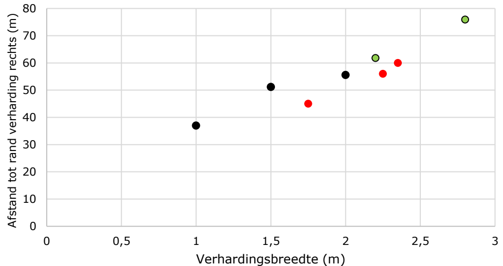
Afbeelding 24. Laterale positie van (solo)fietsers ten opzichte van de rechter rand van het fietspad (Theuwissen, 2021)
