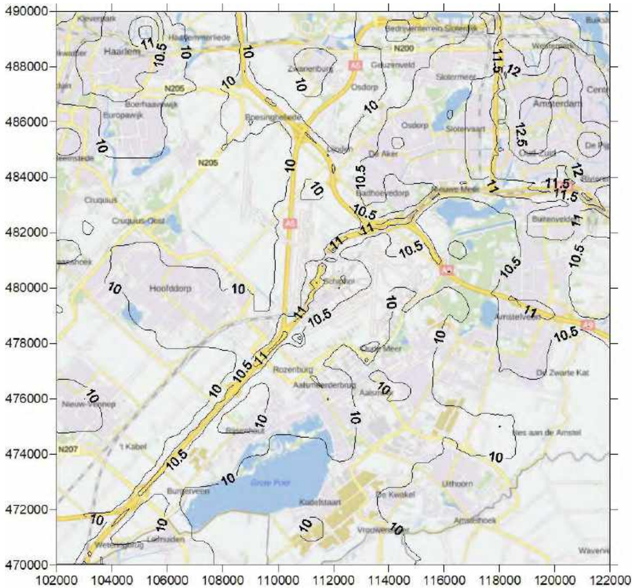
Figuur K.28: Contourplot (20x20 km) van de jaargemiddelde concentratie PM_{2.5} (in \mu g/m^3 ) scenario 450k_HS zichtjaar 2020
