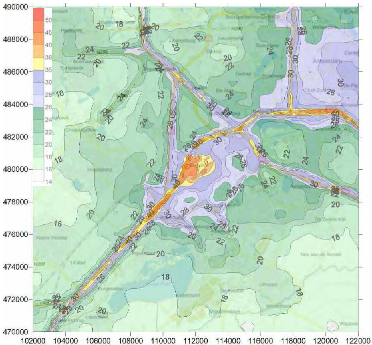
Figuur K.1: Contourplot (20x20 km) van de jaargemiddelde concentratie NO 2 (in µg/m 3 ) scenario 450k_HS jaar 2015
