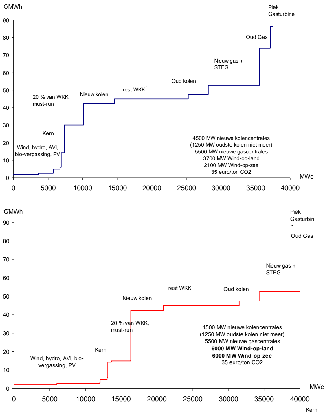
Figuur 2.4 Indicatieve en illustratieve marginale aanbod curves in 2020 (100% beschikbaar en zonder exportvraag). Boven: UR-GE. Beneden: Idem UR-GE, maar dan ter illustratie met windvermogen van 5800 MW tot 12000 MW uitgebreid
