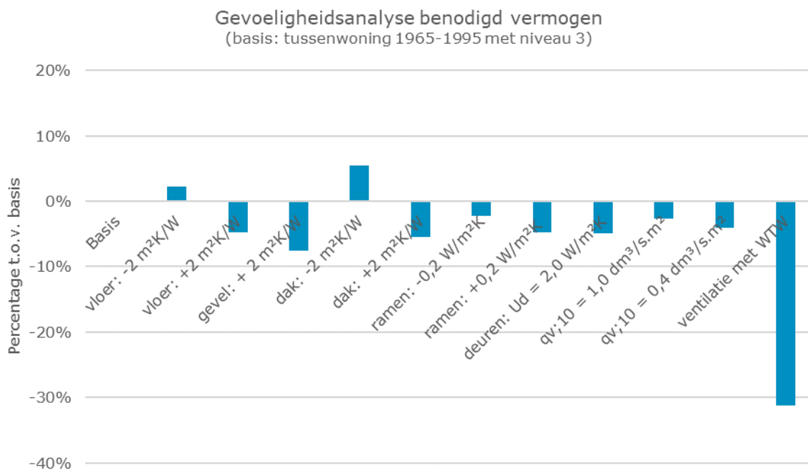
Figuur 29: gevoeligheidsanalyse benodigd verwarmingsvermogen (bouwkundig en ventilatiesysteem)
