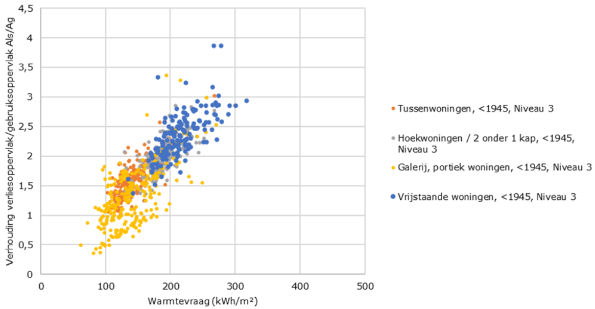
Figuur 61: netto warmtevrage: Bouwperiode tot 1945, niveau 3
