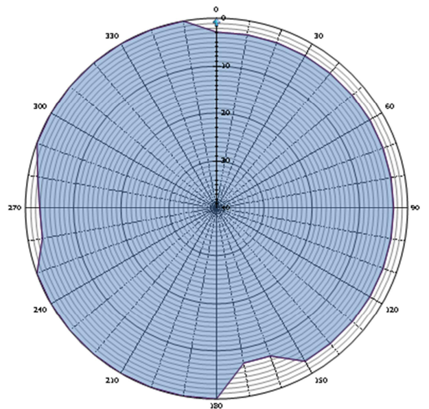
Grafische weergave antennediagram (0 = geografisch)
