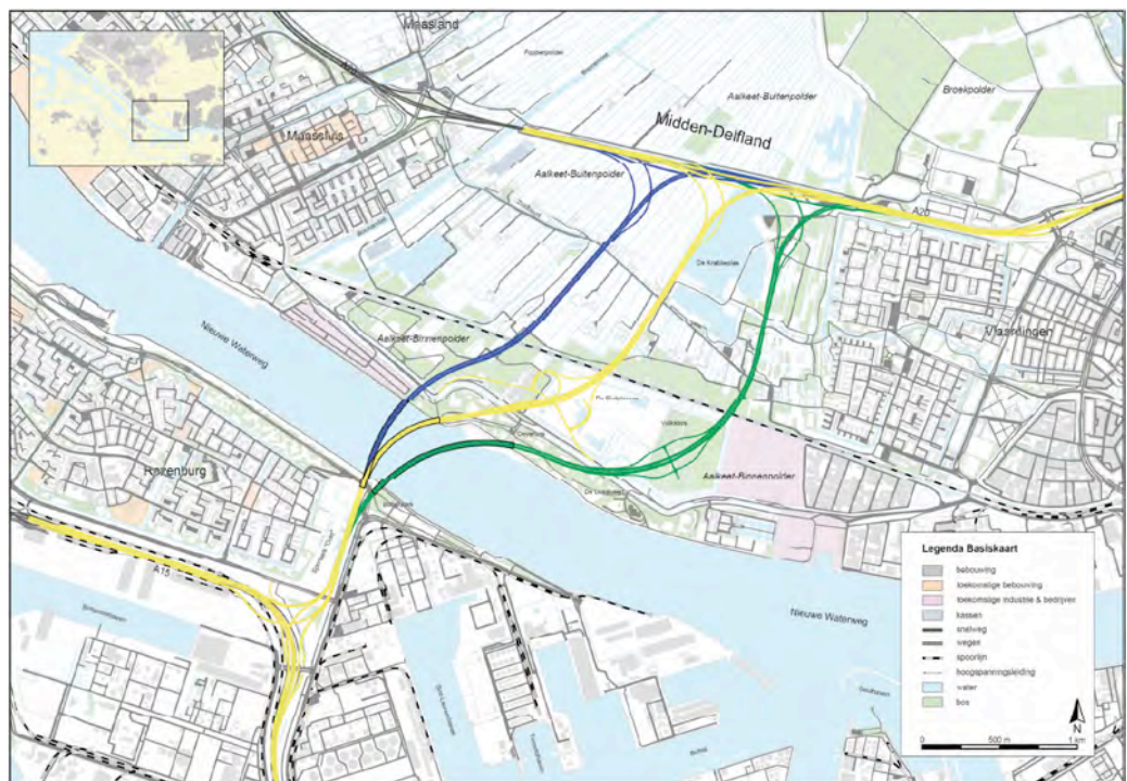
Afbeelding 2.3. Varianten Blankenburgverbinding
