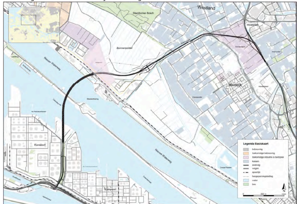
Afbeelding 2.2: Varianten Oranjeverbinding
