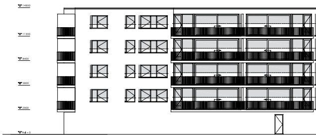
Rechterzijgevel (oost)
