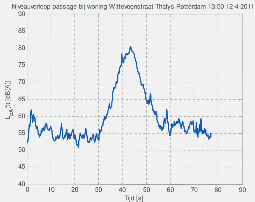
Figuur C4: Niveauperloop van de A-gewogen geluiddruk 2 meter voor de gevel van de woning aan de Witteveenstraat, voor een Thalys passage, richting Rotterdam, op 12 april 2011 om 13:50.
