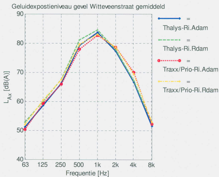
Figuur 6: Spectra van het gemiddelde gemeten geluidexpositieniveau L_{Ax} bij de gevel van de woning aan de Witteveenstraat, van alle gemeten treinpassages per treintype per rijrichting gedurende alle drie meetdagen.
