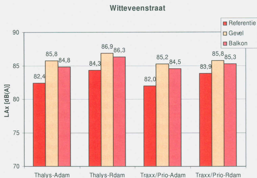
Figuur 5: Gemeten geluidexpositieniveaus L_{Ax} voor de gevel van de woning Witteveenstraat 201, op het balkon en op de referentiepositie, gemiddeld over drie meetdagen, per treintype en rijrichting.
