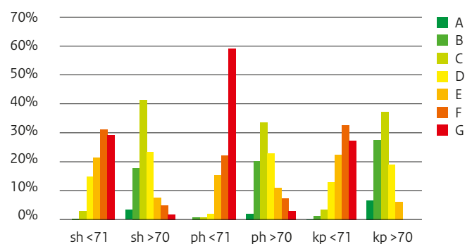
Figuur 4.6 Relatie tussen energielabel, eigendoms-categorie en bouwjaarklasse
