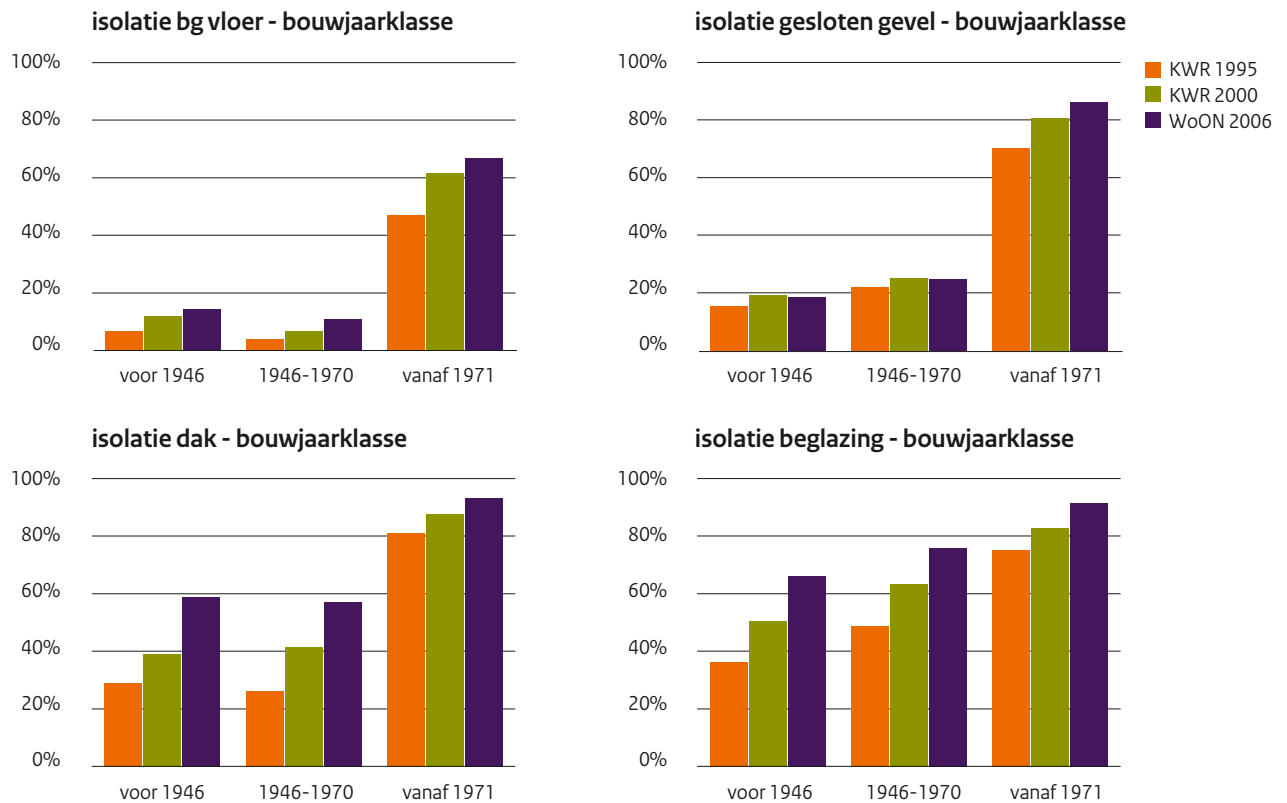
Figuur 5.6 De isolatiegraad van bouwdelen per bouwjaarklasse 4
