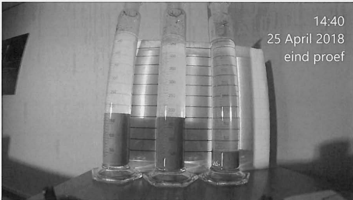
Figuur 5: De toestand 49 uur na het begin van het bezinken. Het bovenstaande water is na 69 uur bezinken met een sifon overgebracht in door Deltares verschafte kunststof flessen voor watermonsters en het vaste stofgehalte van die watermonsters is bepaald.
