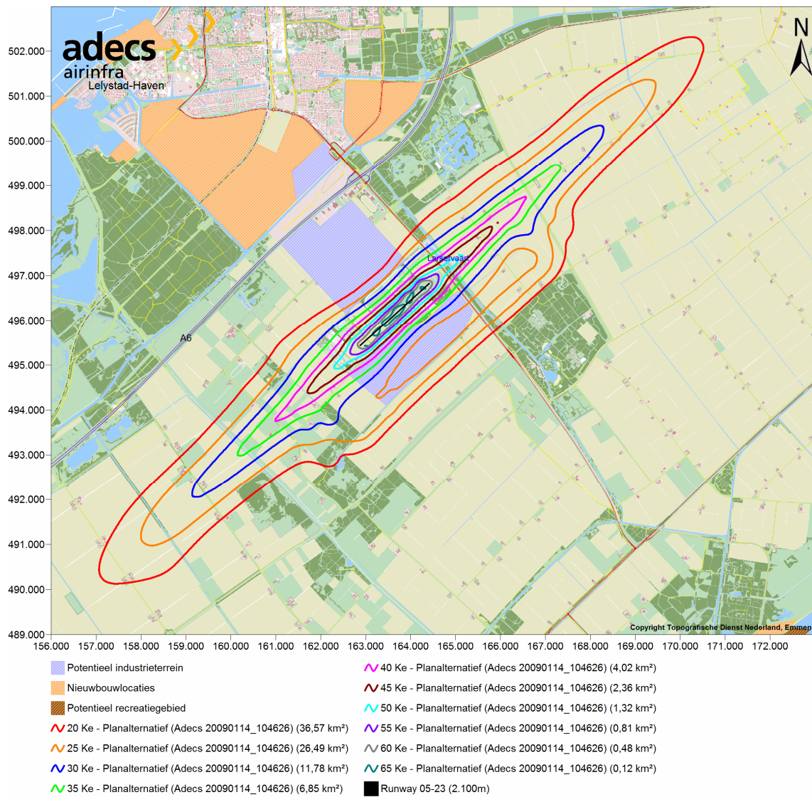
Figuur 30 20 t/m 65 Ke-contouren behorende bij het planalternatief.
