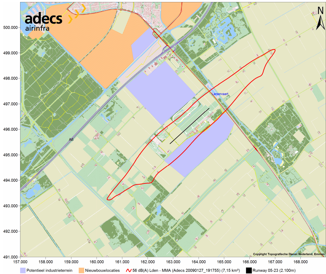
Figuur 44 56 dB(A) L_{den} -contour behorende bij het meest milieuvriendelijke alternatief.
