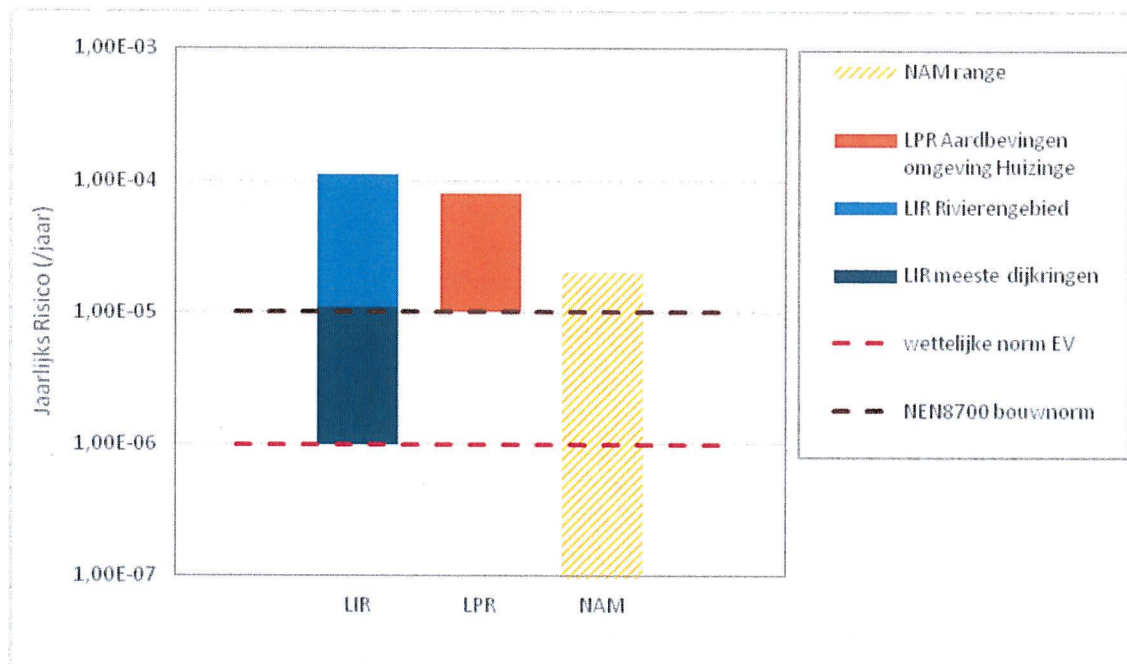
Figuur 1: Het Lokaal Persoonlijk Risico (LPR) voor aardbevingen in de omgeving van Huizinge in relatie tot het Lokaal Individueel Risico (LIR) voor overstromingen, de wettelijke norm voor Externe Veiligheidsinrichtingen (EV) en de NEN 8700 bouwnorm voor belastingen op huizen.
