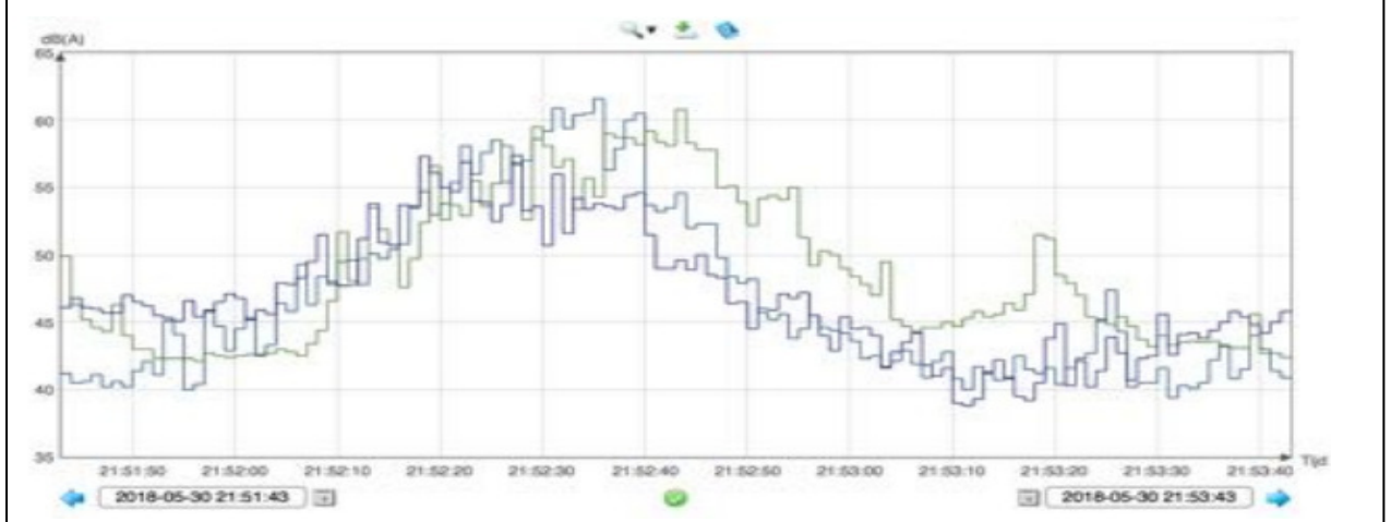
Passage 66: 21:52:43 Biddinghuizen - Park Singel [LASmax= 61,6 dB(A)]
