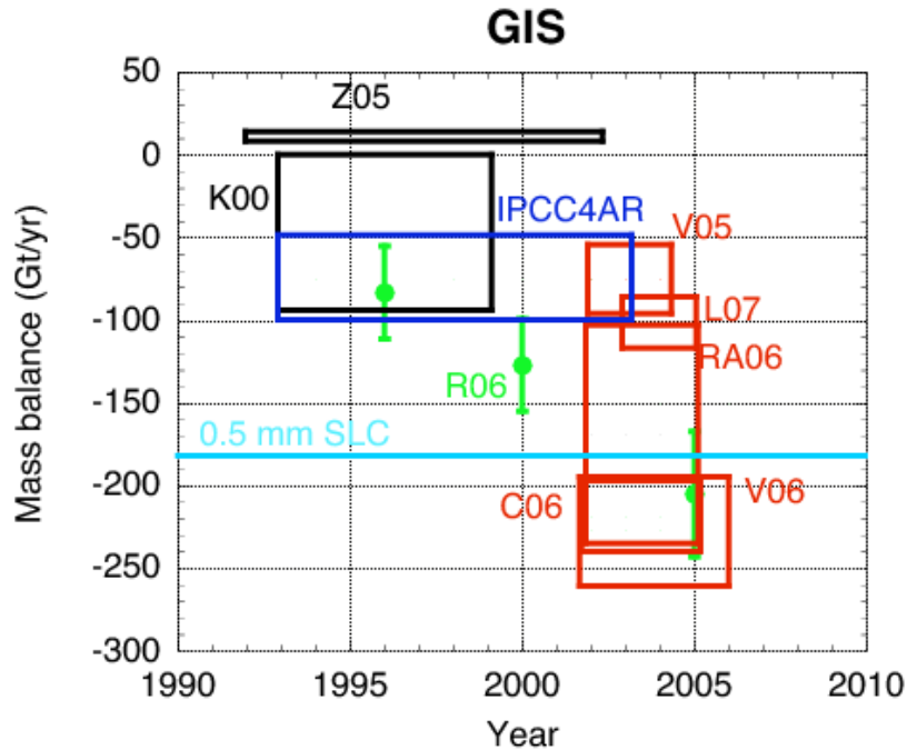
Figuur 1.9: Verschillende schattingen van de massabalans van de Groenlandse ijskap. Groen – Bepaald uit uit Insar metingen van ijsnsnelheid. Rood – zwaartekrachtmetingen (GRACE), zwart - radarhoogtemetingen. Blauw – IPCC AR4 schatting. De cijfers corresponderen met het jaar van publicatie, de letter met de naam van de eerste auteur. De schatting van IPCC is gebaseerd op Z05, K00, V05, R06, C06 Z05 (Zwally et al. 2005), K00 (Krabill et al. 2000), R06 (Rignot en K 06), C06 (Chen et al. 2006), V06 (Velicogna et al. 2006), RA06 (Ramilien et al. 2006).
