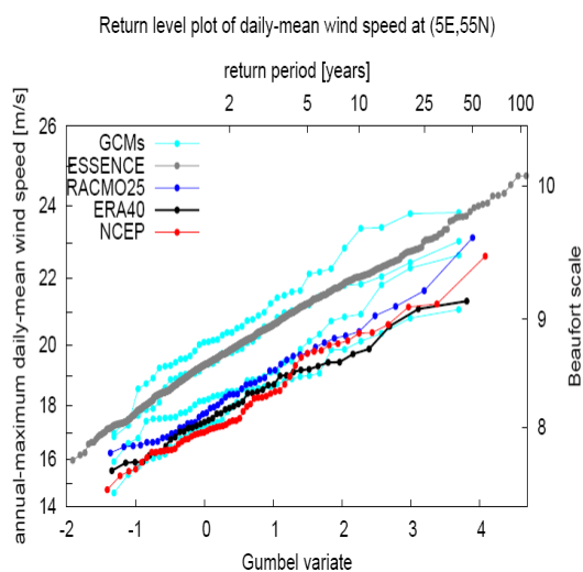
Figuur 2.5. Gumbel grafiek van jaarlijkse maximum windsnelheid op 5^{\circ}\text{O} , 55^{\circ}\text{N} . De blauwgroene GCMs-gelabelde lijnen verwijzen naar de vier mondiale klimaatmodellen die gebruikt zijn in de KNMI'06 scenario's (KNMI 2006) en de blauwe RACMO25 gelabelde lijn naar een run met het regionale klimaatmodel RACMO met een resolutie van 25 km, op basis van ERA-40 grensvoorwaarden. Waarden uit de ERA-40 en de NCEP/NCAR heranalyses zijn weergegeven door respectievelijk zwarte en rode symbolen.
