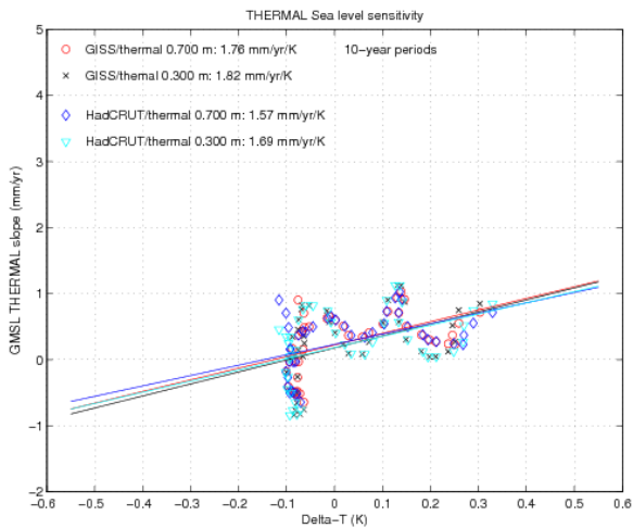
Figuur 1.15: Waargenomen cijfer van thermische uitzetting als een functie van temperatuurstijging, en fits voor thermotherische gevoeligheid van de zeespiegel op basis van waarnemingen (met dank aan Catia Domingues, CSIRO)
