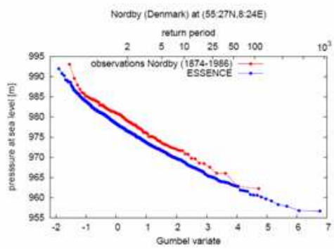
Figuur 2.6: Gumbel grafiek van jaarlijkse minimum luchtdruk op zeeniveau in Nordby, Denemarken ( 8.2^{\circ}O , 55.3^{\circ}N ; links), en wind- en drukvelden voor de situatie die leidt tot de hoogste stormvloed in Hoek van Holland zoals die zich voordeed in de Essence-WAQUA/DCSM98 verzameling (rechts).
