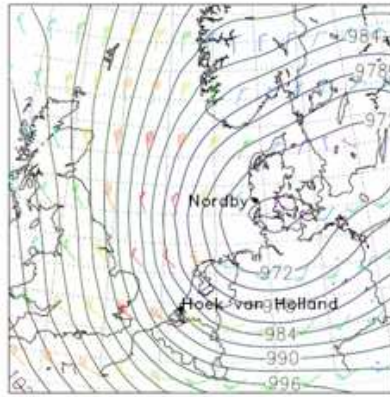
Figuur 2.6: Gumbel grafiek van jaarlijkse minimum luchtdruk op zeeniveau in Nordby, Denemarken ( 8.2^{\circ}O , 55.3^{\circ}N ; links), en wind- en drukvelden voor de situatie die leidt tot de hoogste stormvloed in Hoek van Holland zoals die zich voordeed in de Essence-WAQUA/DCSM98 verzameling (rechts).
