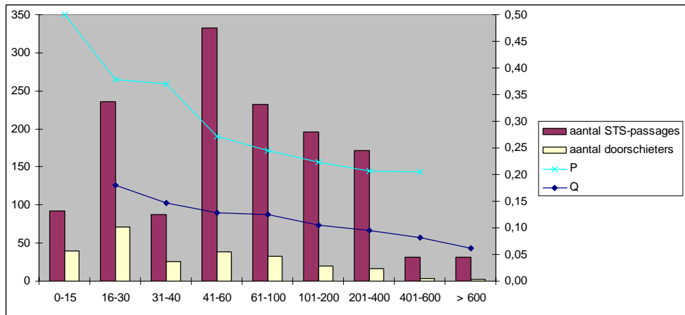
Figuur B9.2 De waarden p en q als functie van de afstand tussen sein en gevaarpunt
