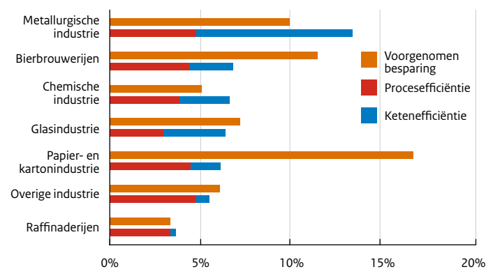
Figuur 2.3 - Maximale voorgenomen besparing voor 2013-2016 versus de gerealiseerde besparing per sector, percentage ten opzichte van het eigen energiegebruik
