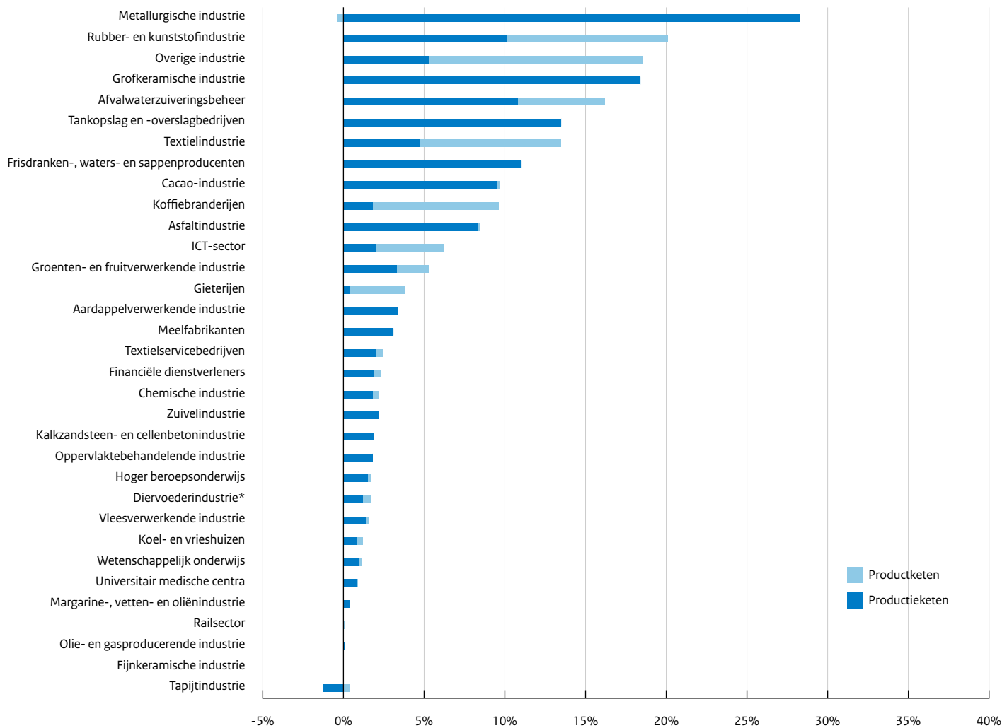
Figuur 3.7 - Besparing per MJA3-sector door efficiëntie in productie- en productketen sinds 2005, gerelateerd aan het eigen energiegebruik
