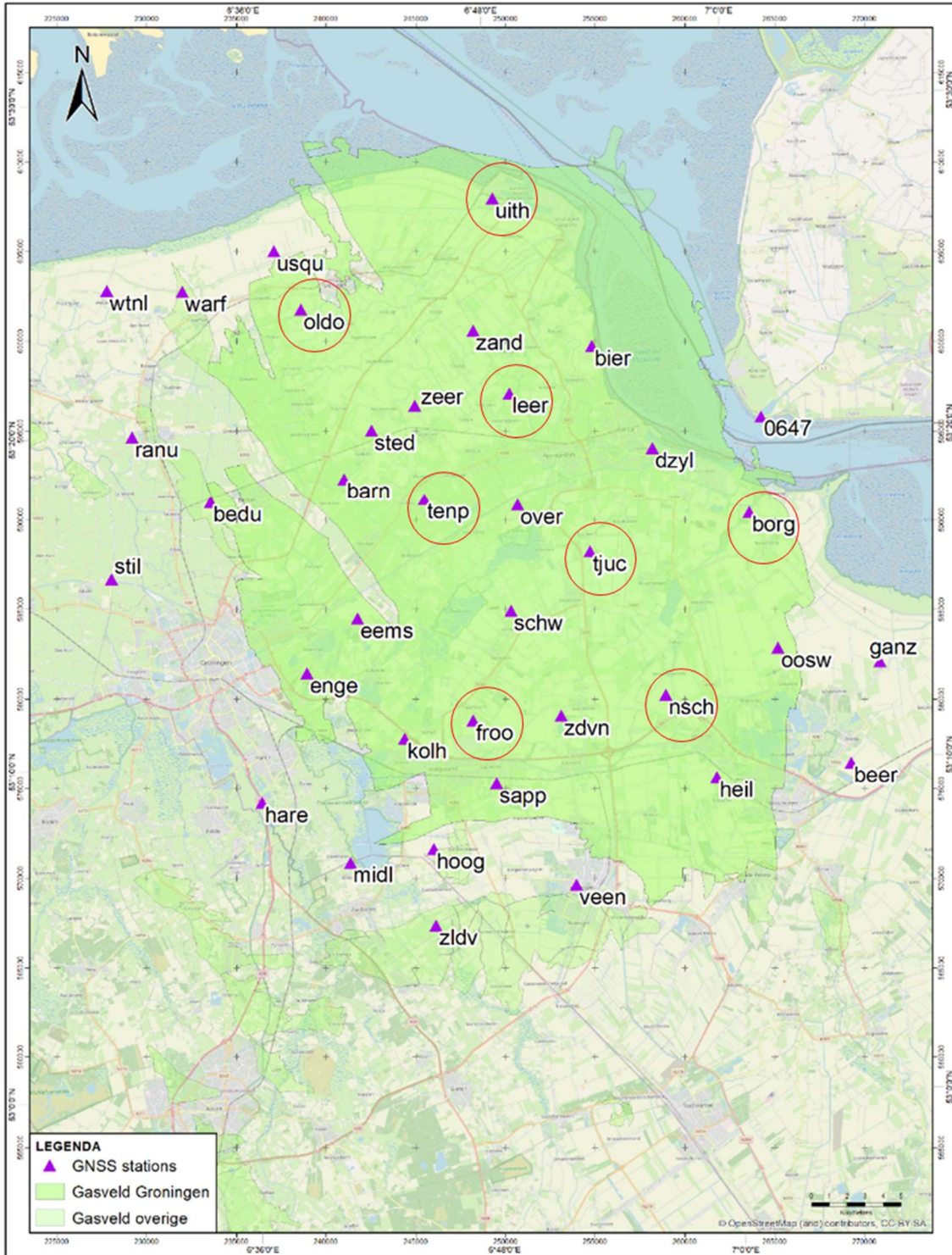
Figuur 6 Kaart met daarop aangegeven de locaties van geïnstalleerde GNSS meetstations boven en rondom het Groningenveld. Van de rood omcirkelde stations zijn in figuur 7 de tijdseries getoond van zowel de gemeten bodemdaling als de gemodelleerde daling
