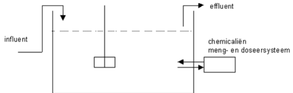
Figuur 18. Schematische weergave precipitatieproces [Emis-Vito, h].
