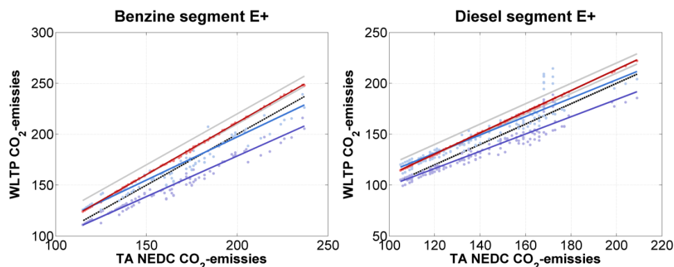
Figuur 5: Relaties tussen NEDC en WLTP emissies voor benzine- en dieselveertuigen afgeleid op basis van de drie verschillende methoden behandeld in paragraaf 3.2.1, 3.2.2 en 3.2.3.
