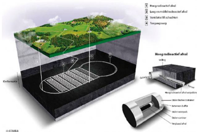
Figuur E.3 Artist's impression van het eindbergingsconcept in Boomse klei (OPERA).
