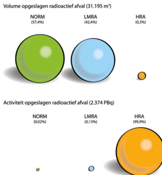
Figuur 3.4 Activiteit en volume van radioactief afval bij COVRA.
