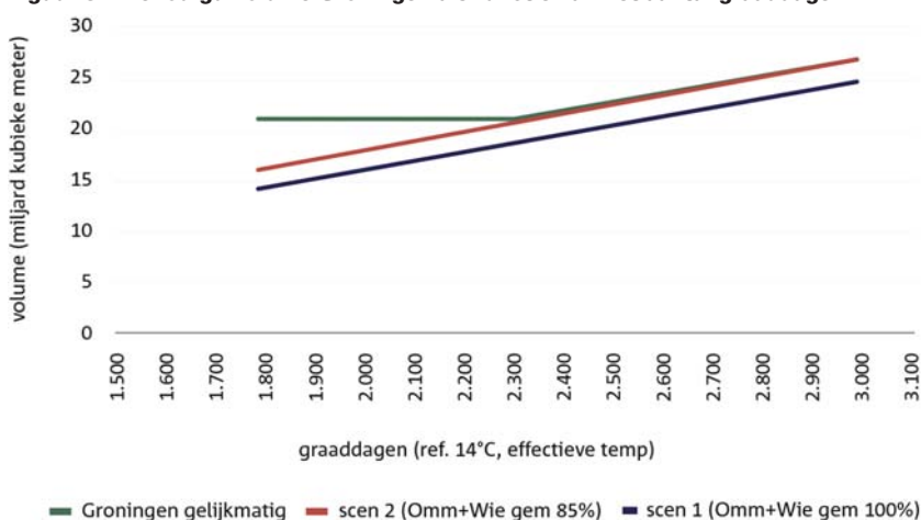
Figuur 8.2 Benodigd volume Groningen als functie van het aantal graaddagen
