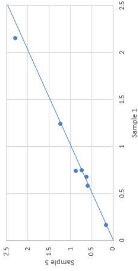
6:2 FTS
