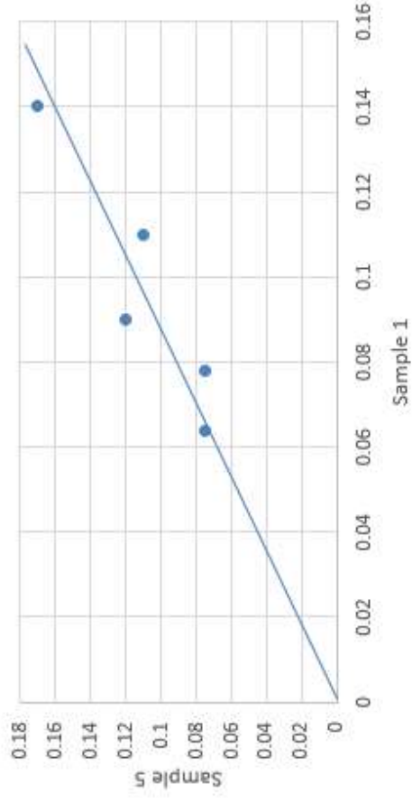
PFBS
